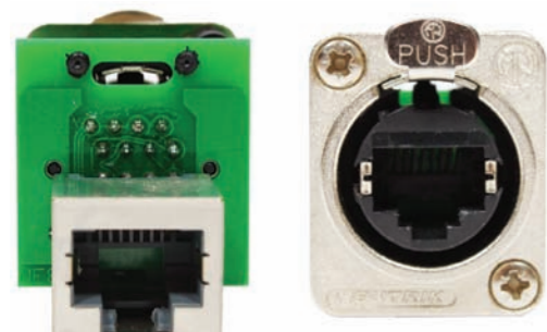
Гнезда RJ – установленное на печатную плату и для установки на панель прибора
